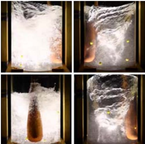
Снимка от провежданите експерименти от Валтер Стапунг
